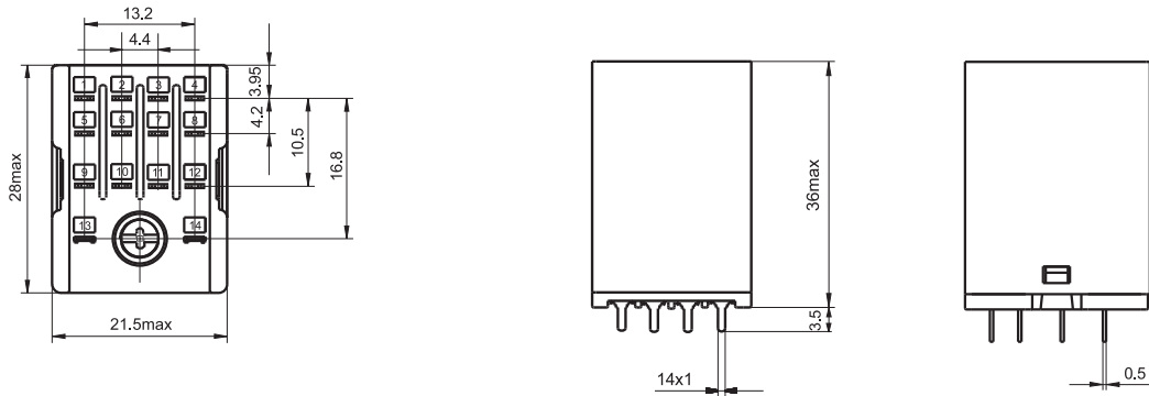
HF18FF-□/□□-4Z2□□□□
